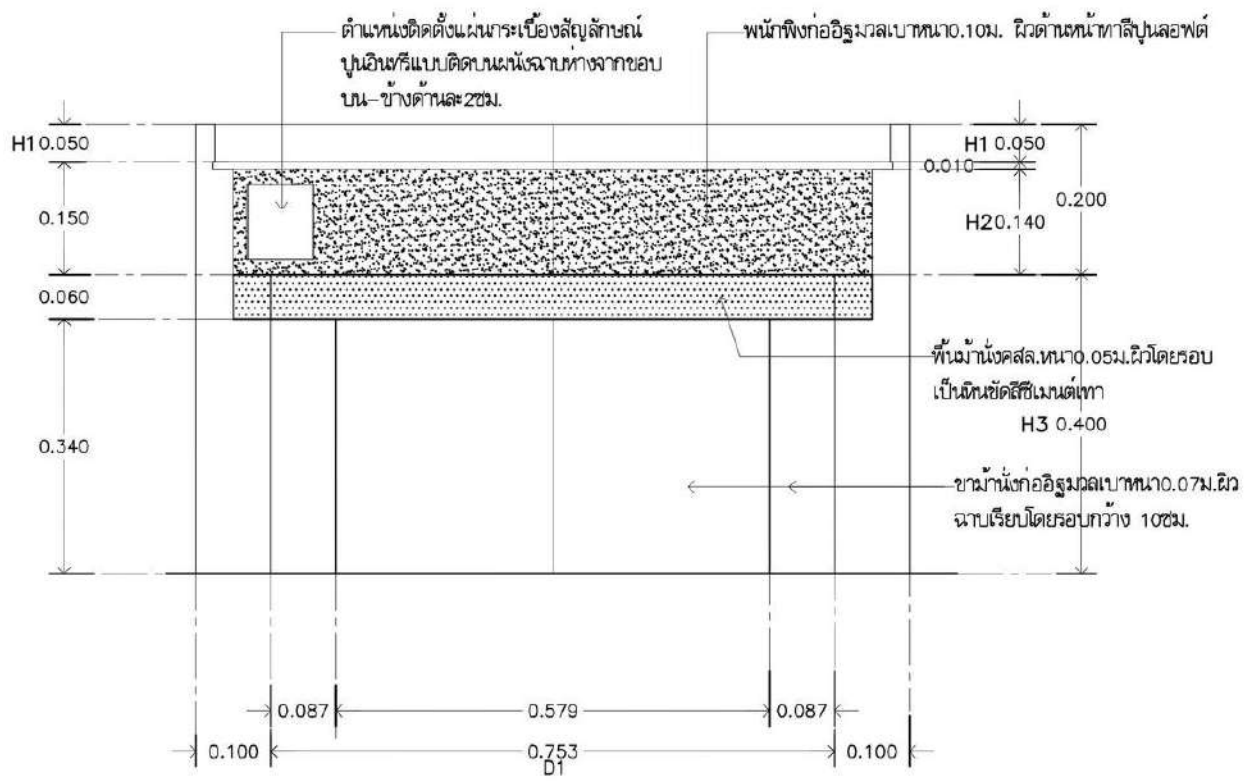
รูปด้านหน้าที 1-1 มาตราส่วน 1:10
