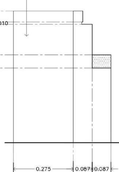
รูปด้านข้างที 4-4 มาตราส่วน 1:10
