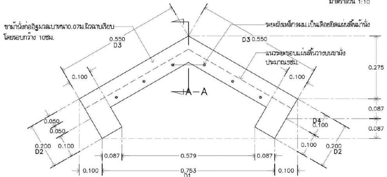
ผังขาม้านั่ง มาตราส่วน 1:10
