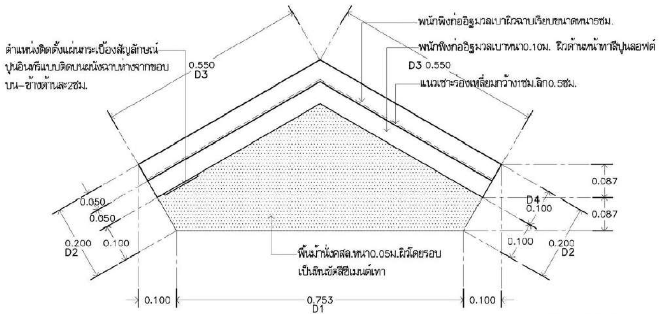
TOP VIEW มาตราส่วน 1:10
